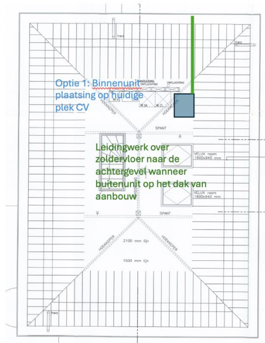
Afbeelding 6: Tekening zolder
