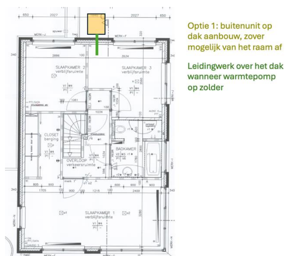
Afbeelding 8: Tekening eerste verdieping
