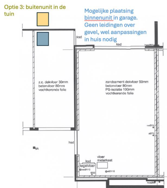
Afbeelding 10: Buitenunit tegen de garage
