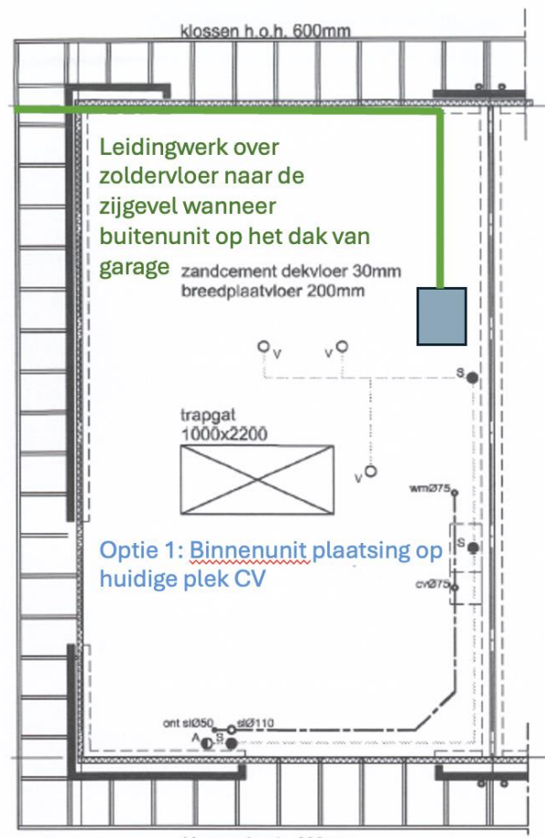
Afbeelding 6: Binnenunit op zolder
