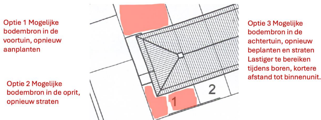
Afbeelding 9: Tekening perceel met mogelijkheden voor bodembron
