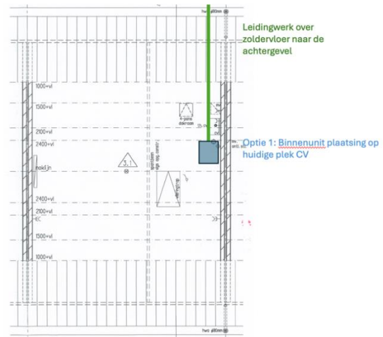
Afbeelding 6: Tekening zolder
