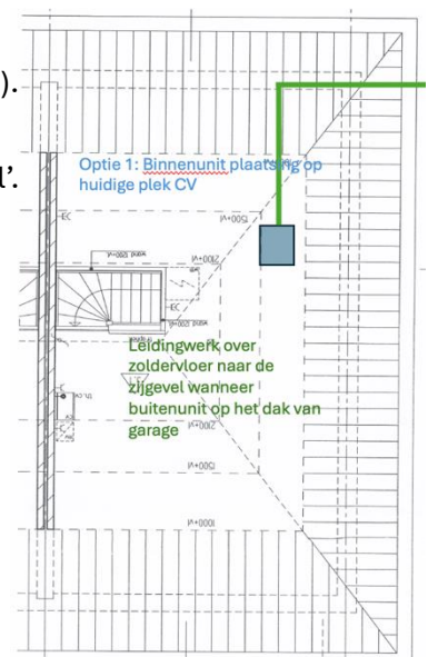
Afbeelding 6: Tekening zolder
