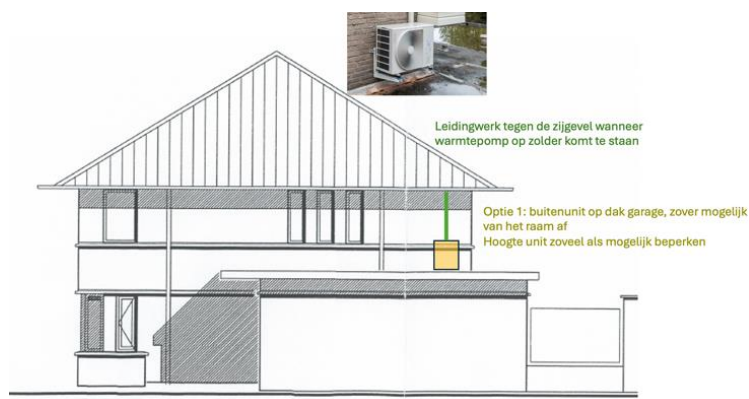
Afbeelding 7: Tekening zijgevel
