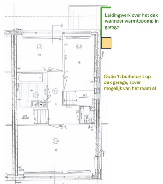
Afbeelding 8: Tekening eerste verdieping
